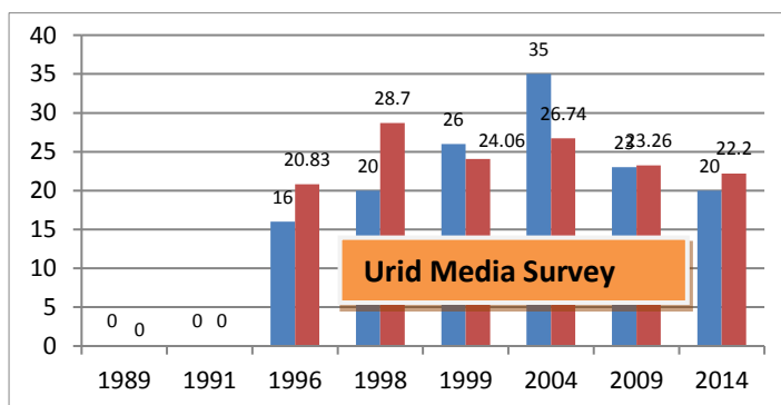
SP 1989-2014
